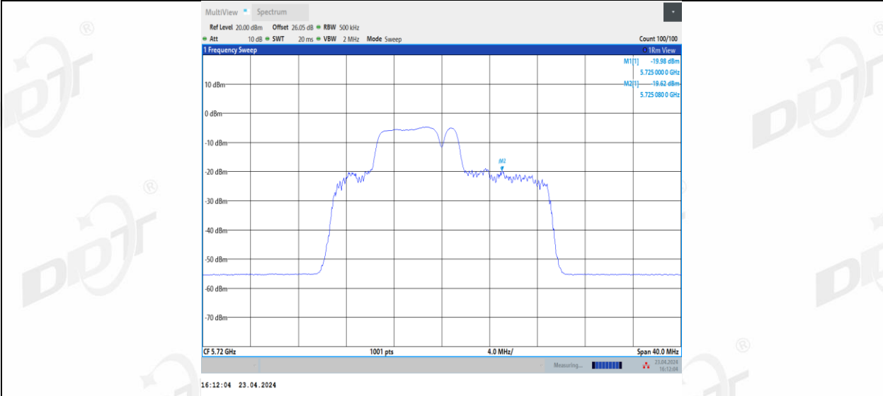
11BE20MIMO_Ant1_5720_UNII-3_52+26_3
