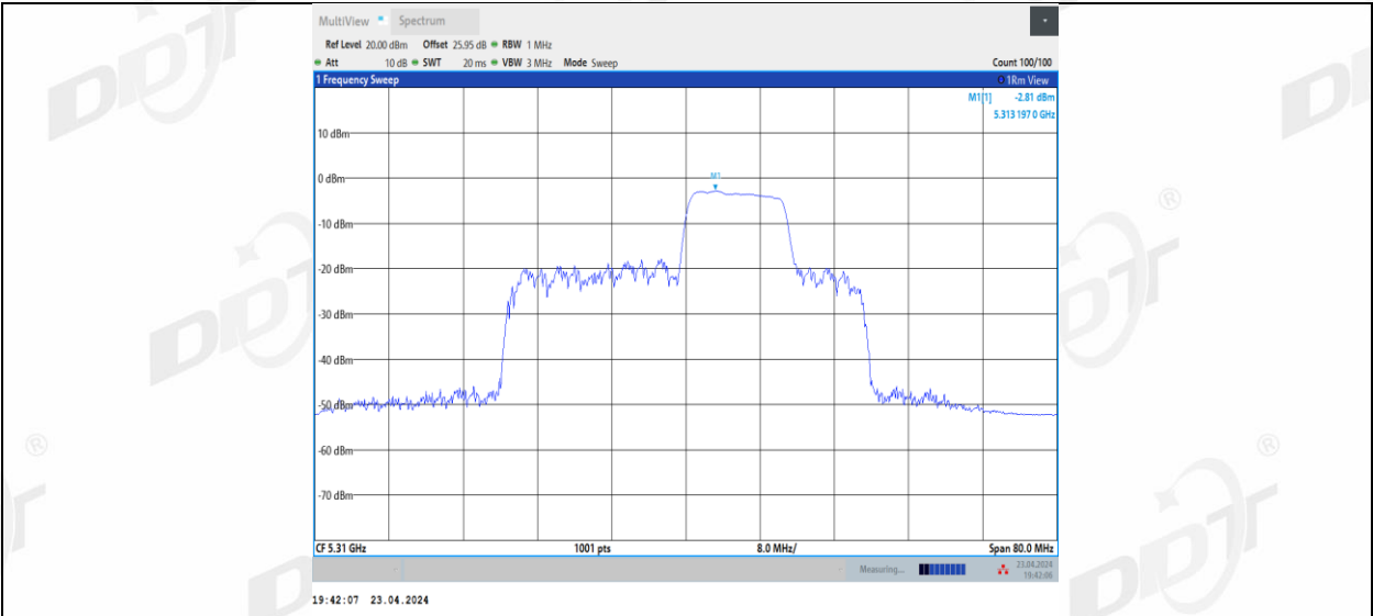
11BE40MIMO_Ant1_5310_106+26_4
