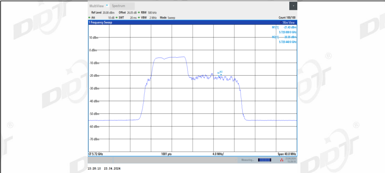
11BE20MIMO_Ant1_5720_UNII-3_52+26_2
