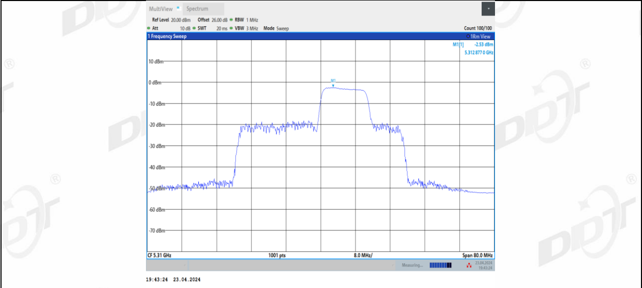
11BE40MIMO_Ant2_5310_106+26_4
