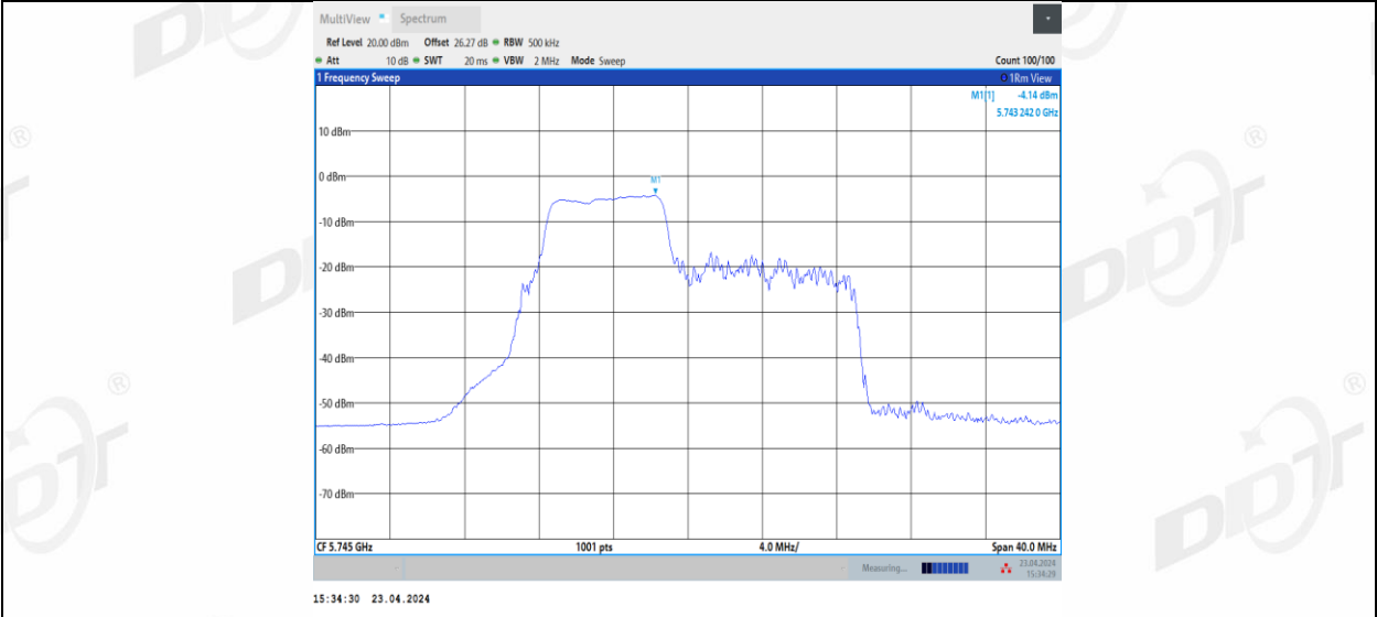
11BE20MIMO_Ant2_5745_52+26_2
