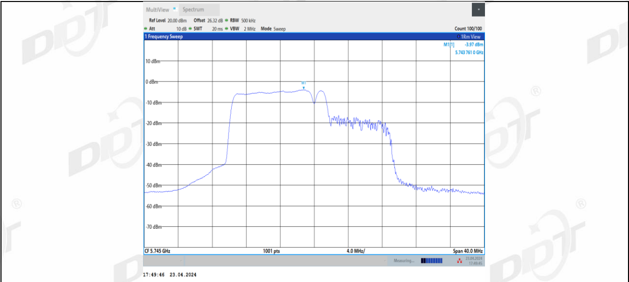
11BE20MIMO_Ant1_5745_106+26_2
