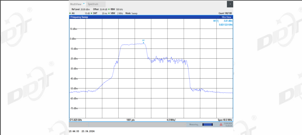
11BE20MIMO Ant3 5825 52+26 2
