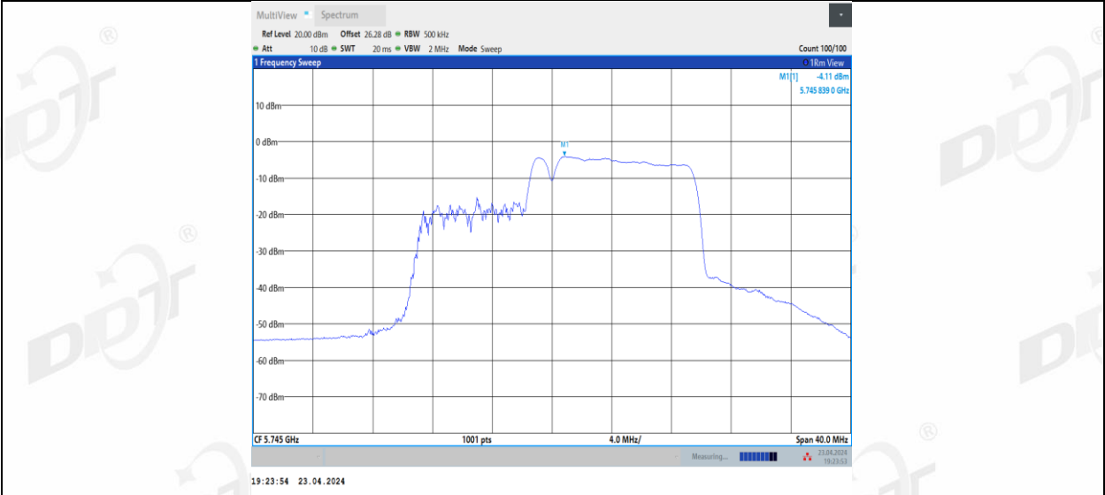
11BE20MIMO_Ant2_5745_52+26_1
