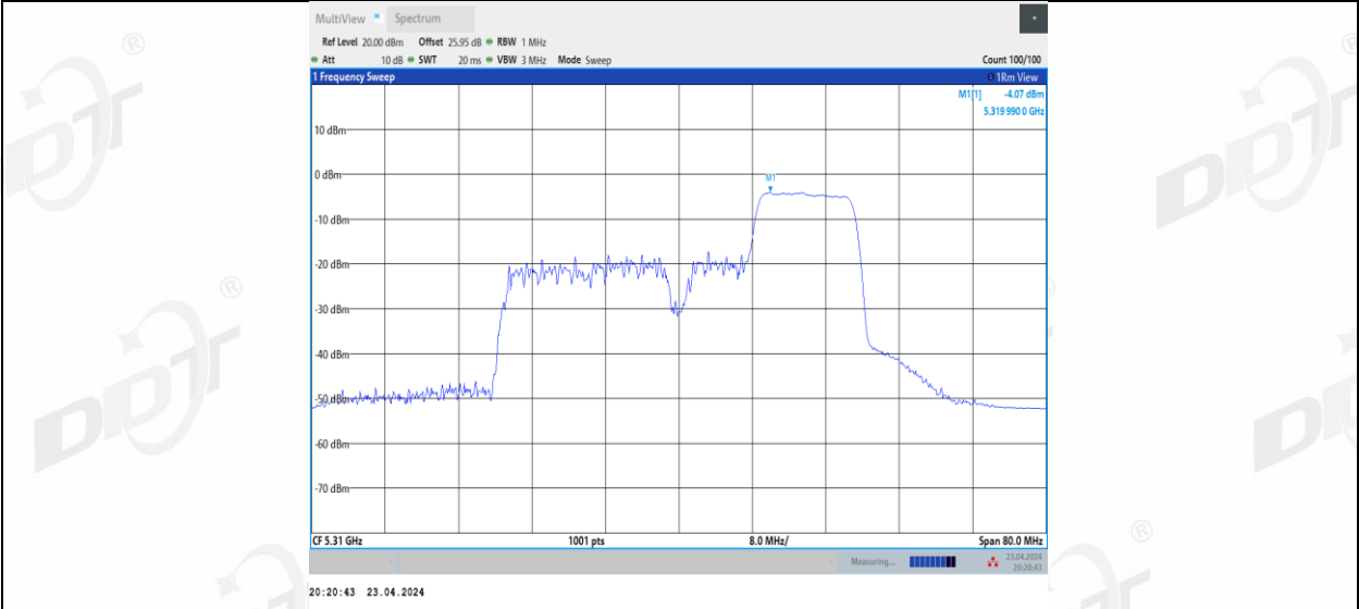
11BE40MIMO_Ant2_5310_106+26_3
