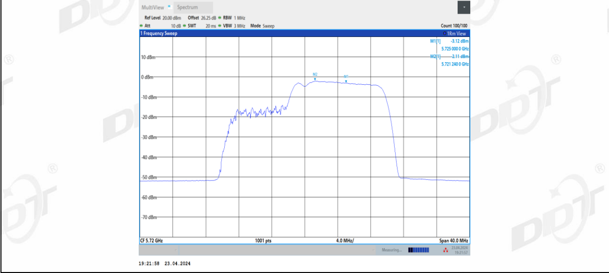
11BE20MIMO Ant1 5720 UNII-3 52+26 1
