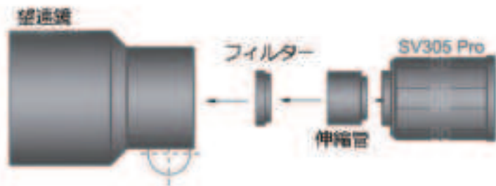
接続望遠鏡
