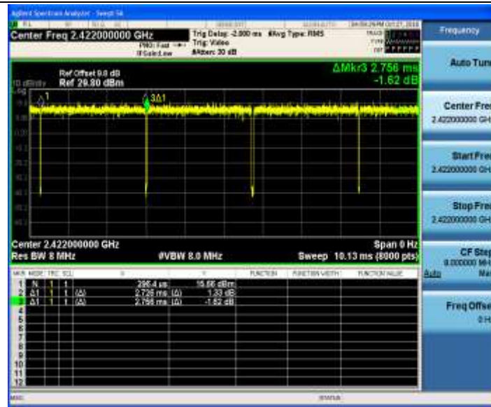
11G_Ant2_2422
