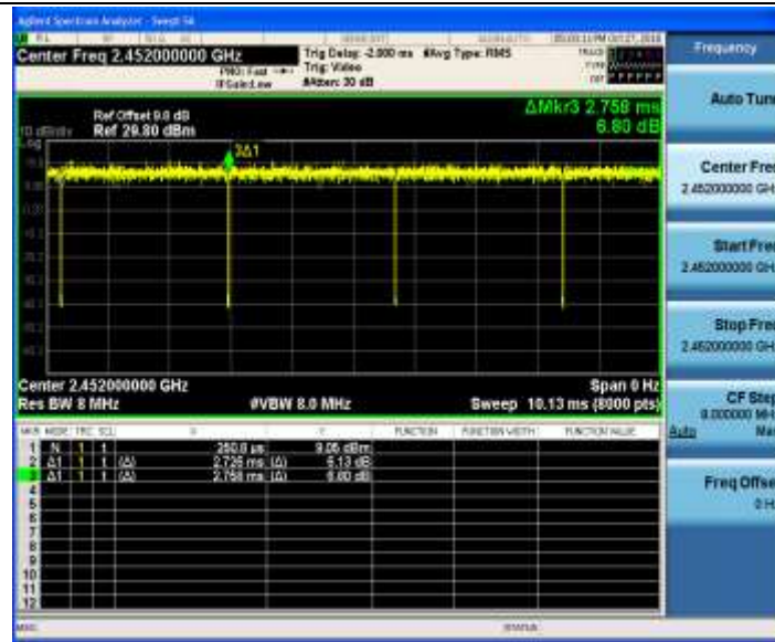
11G_Ant2_2452
