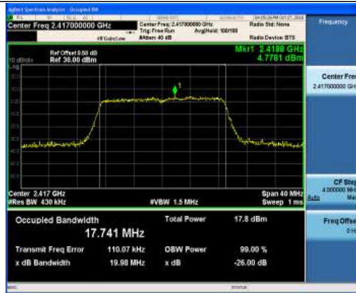
11N20MIMO_Ant2_2417
