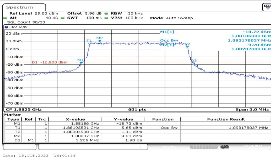
Band25-1.4MHz-QPSK-26365-6RB#0-PASS
