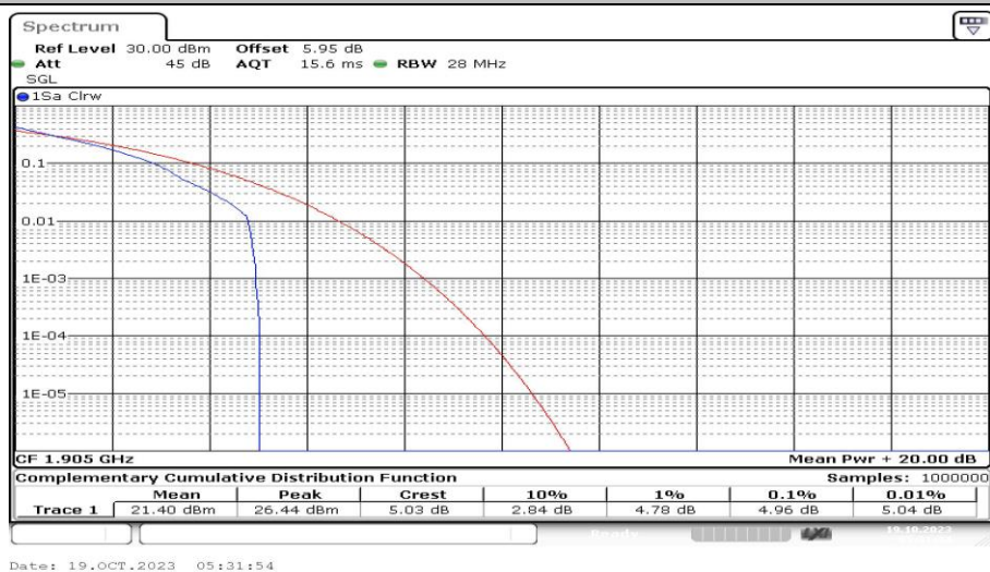
Band25-20MHz-QPSK-26590-1RB#0-PASS
