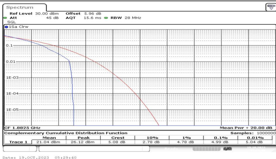
Band25-20MHz-QPSK-26365-1RB#0-PASS
