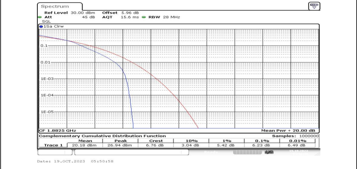
Band25-10MHz-16QAM-26365-25RB#0-PASS
