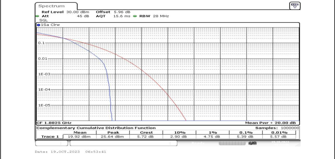
Band25-20MHz-16QAM-26365-25RB#0-PASS
