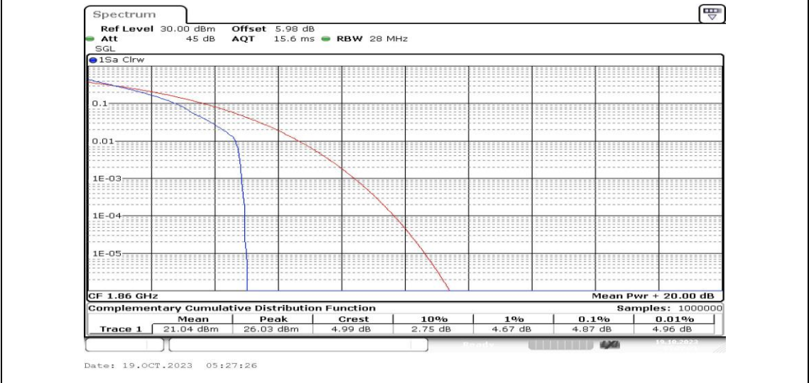
Band25-20MHz-QPSK-26140-1RB#0-PASS
