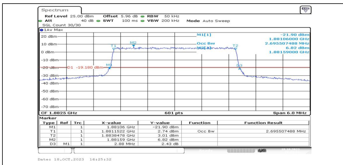
Band25-3MHz-QPSK-26365-15RB#0-PASS
