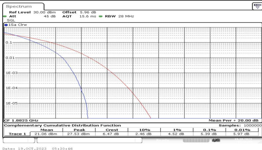
Band25-20MHz-QPSK-26365-100RB#0-PASS
