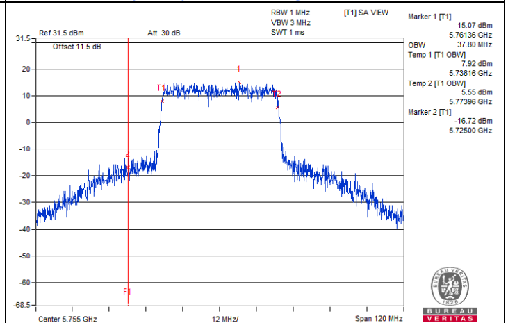
802.11ax (HE40) Beamforming / Chain 1 : CH 151
