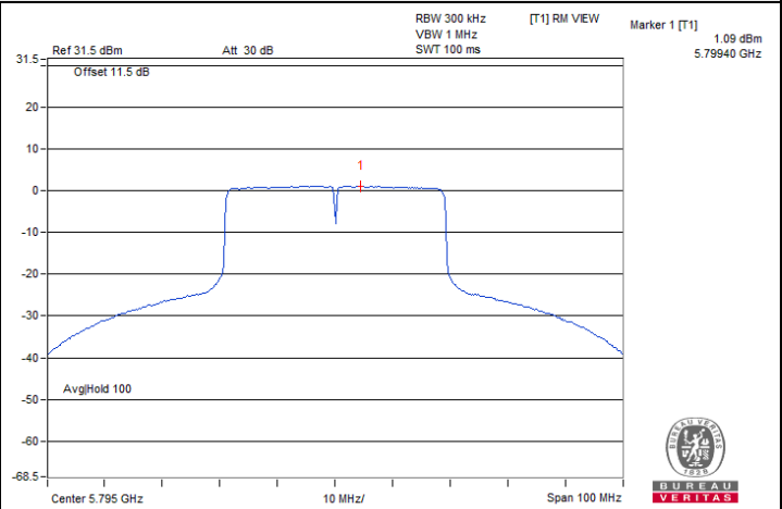
802.11ax (HE40) Beamforming / Chain0 : CH 159
