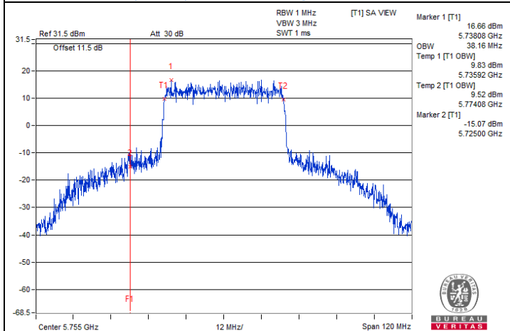
802.11ax (HE40) Beamforming / Chain 0 : CH 151
