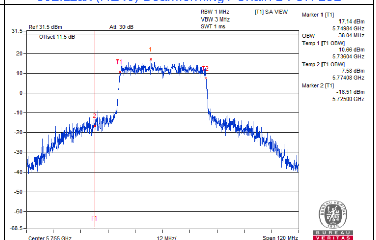
802.11ax (HE40) Beamforming / Chain 3 : CH 151
