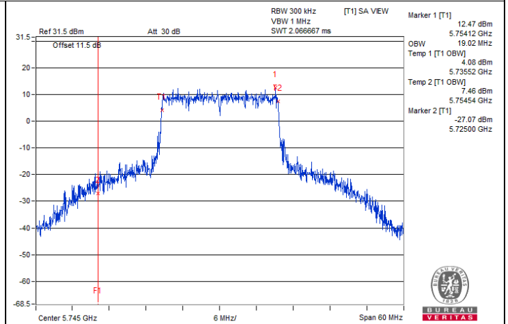
802.11ax (HE20) Beamforming / Chain 3 : CH 149
