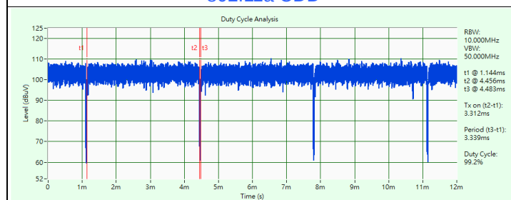
802.11ax (HE40) CDD
