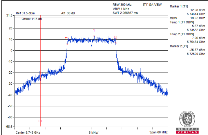
802.11ax (HE20) Beamforming / Chain 2 : CH 149
