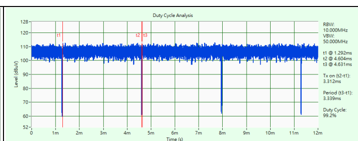
802.11ax (HE20) CDD
