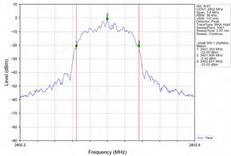
PI/4DQPSK 2DH5 LCH 2402MHz Ant1 NTN
