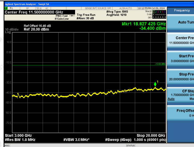
3 GHz~20 GHz
