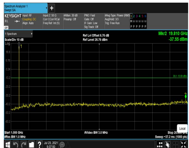
Band2-1.4MHz-QPSK-19193:1000~20000MHz
