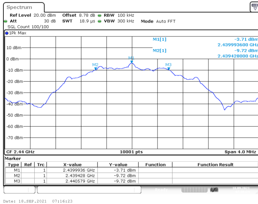
-6dB Bandwidth NVNT BLE 2M 2440MHz Ant1
