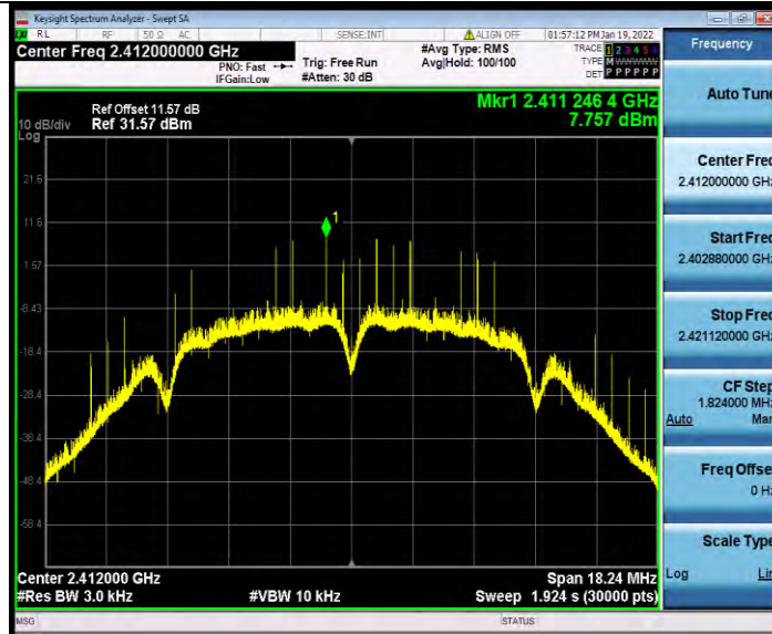
11B_Ant1_2412
