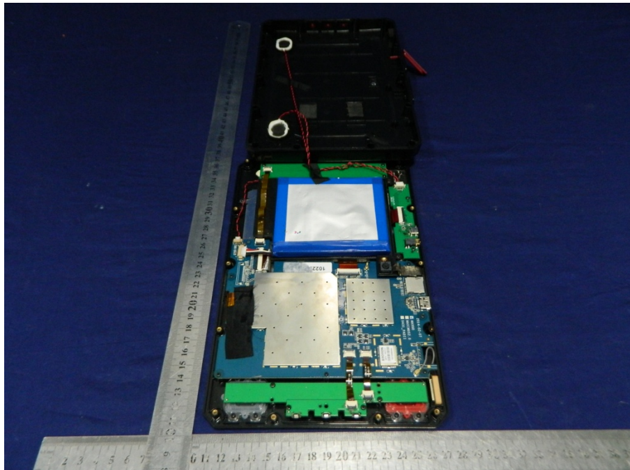
GPS Antenna
