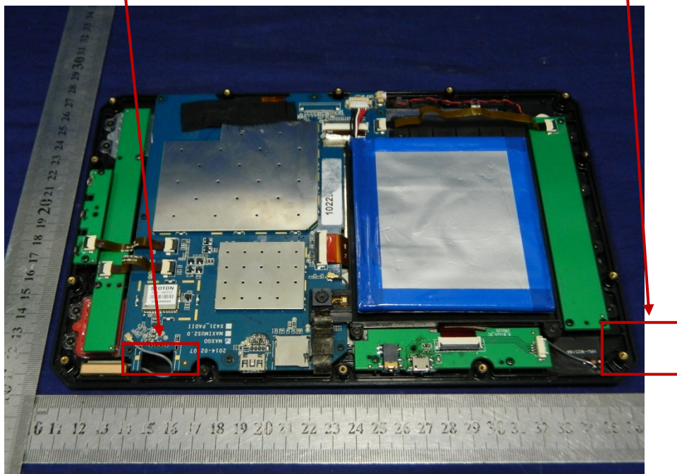
GPS Antenna
