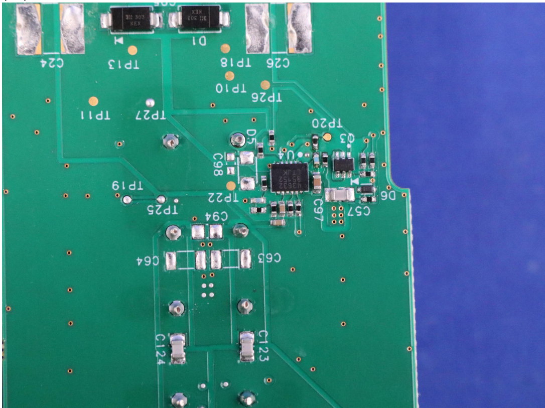
(13) EUT Photo
