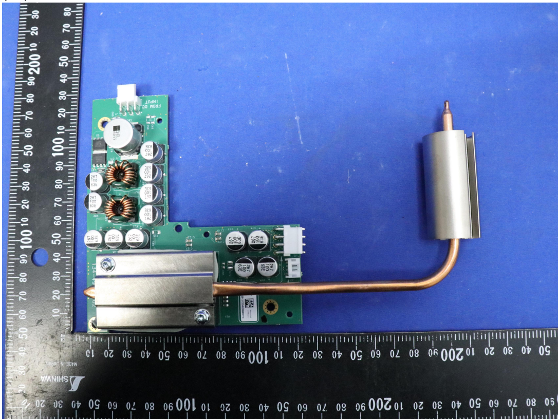
(13) EUT Photo
