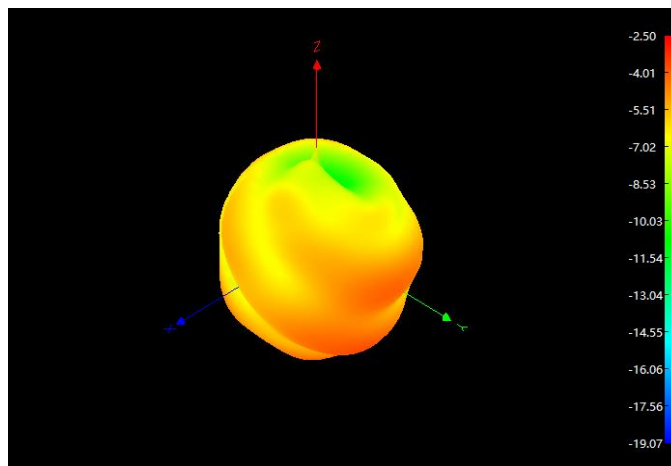
2500MHz 3D
