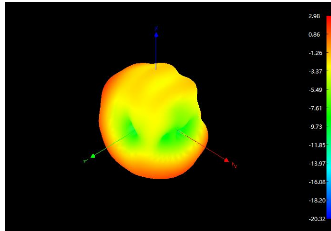
2450MHz 3D
