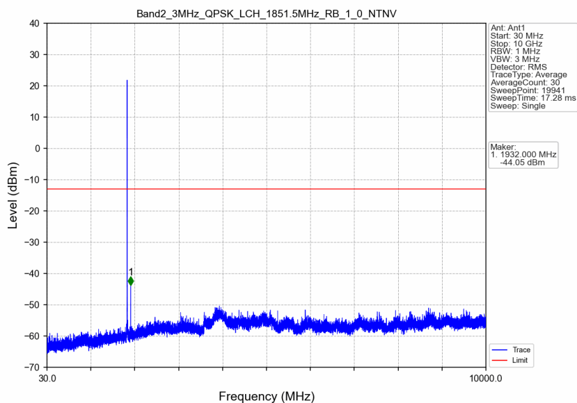
Band2_3MHz_QPSK_LCH_1851.5MHz_RB_1_0_NTNV
