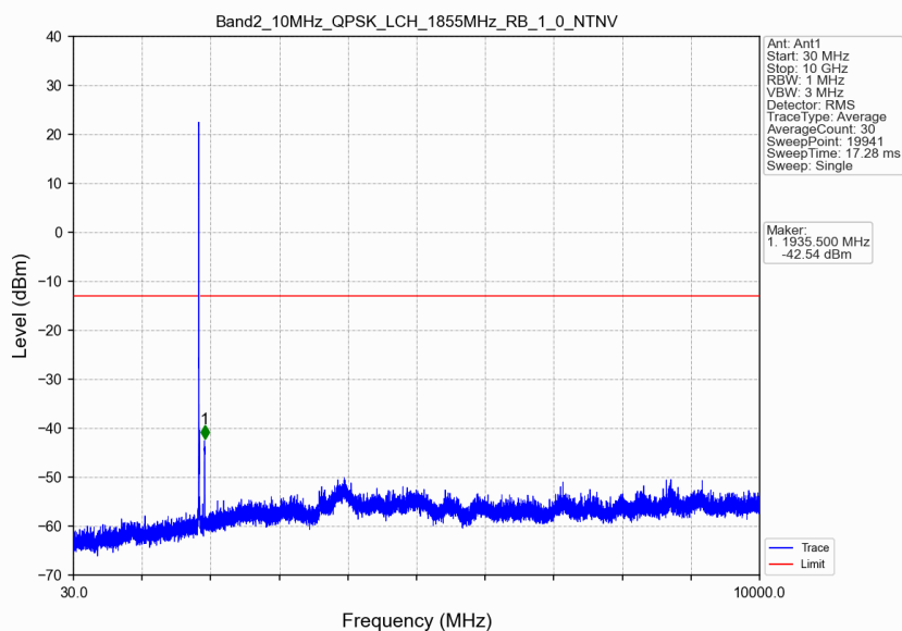
Band2_10MHz_QPSK_LCH_1855MHz_RB_1_0_NTNV
