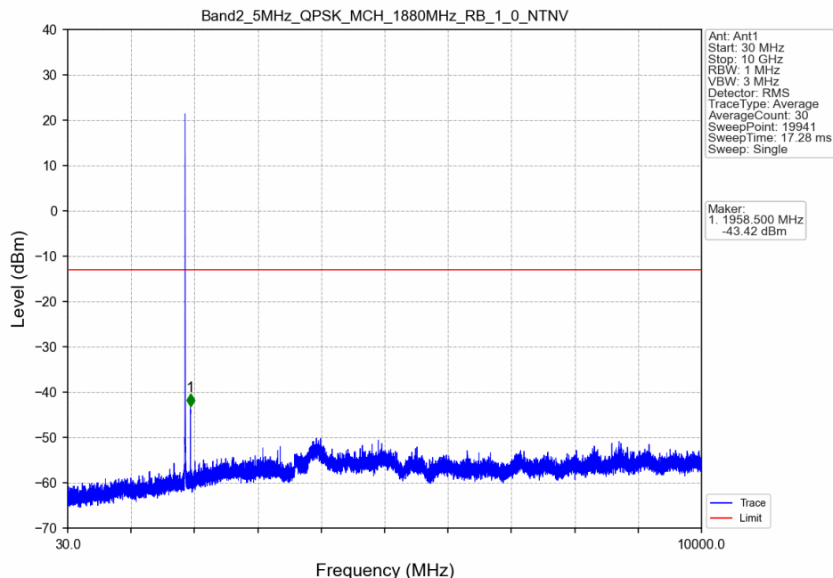
Band2_5MHz_QPSK_MCH_1880MHz_RB_1_0_NTNV
