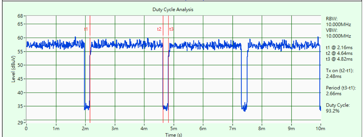
802.11n (HT40)
