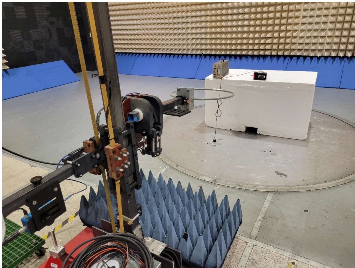
RSE 10kHz – 30MHz
