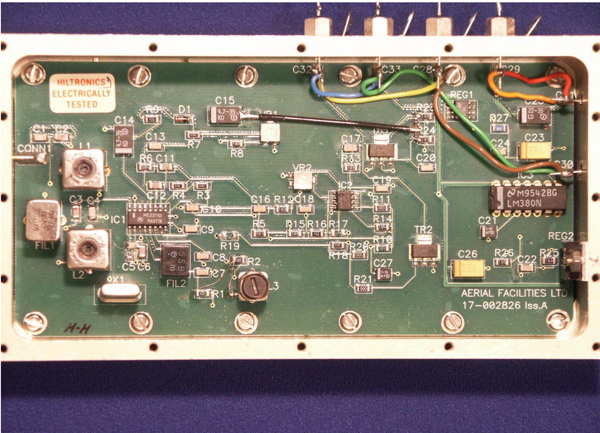
17-002802 (Simplex Rx/Squelch)
