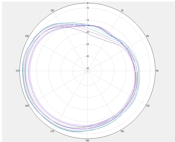
GSM850 / WCDMA B5 / LTE B5 \Theta=90\text{deg}
