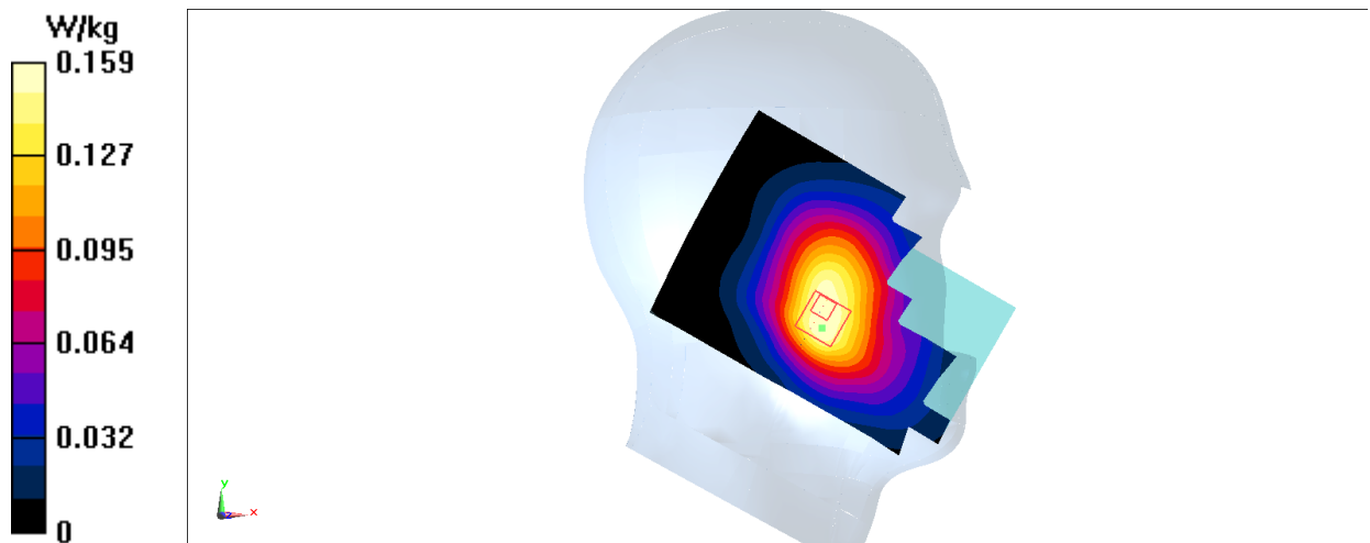
Fig.5 WCDMA 850
