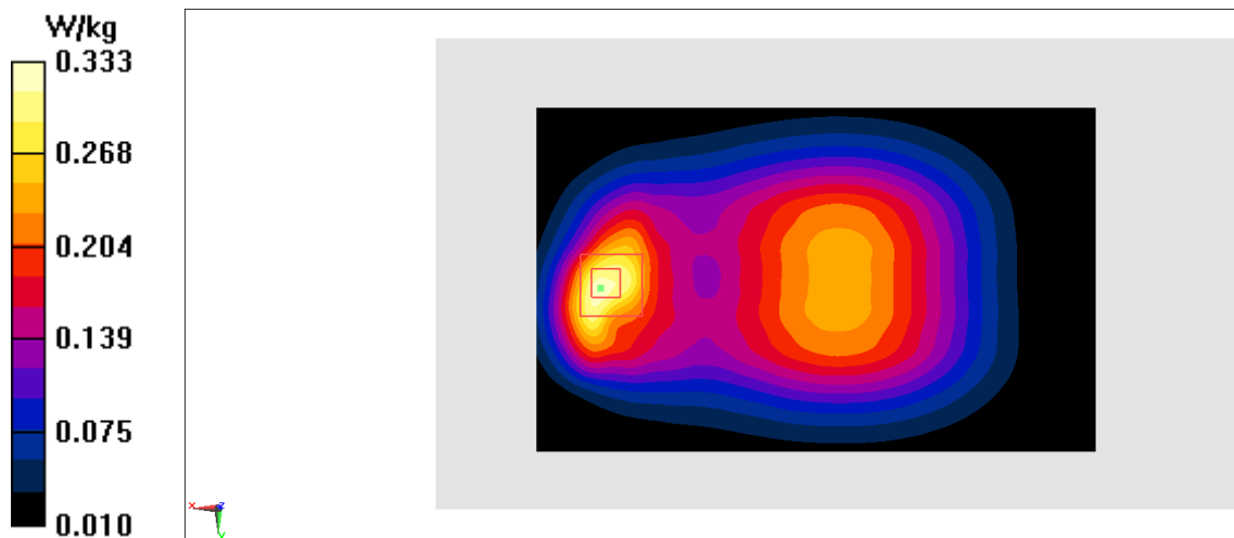
Fig.6 WCDMA 850
