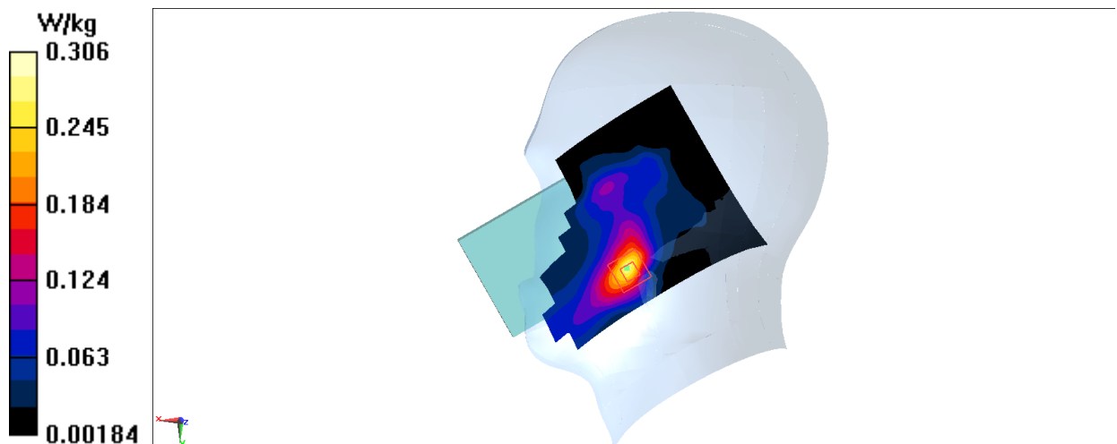
Fig.9 LTE Band7
