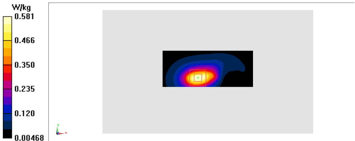
Fig.10 LTE Band7
