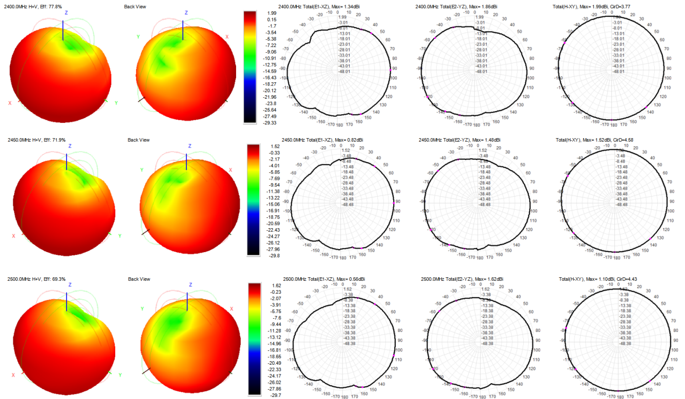
天线场型图
