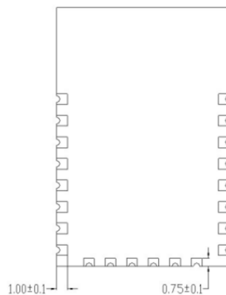
背面
