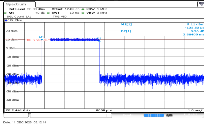
3DH5_Ant1_Hop
