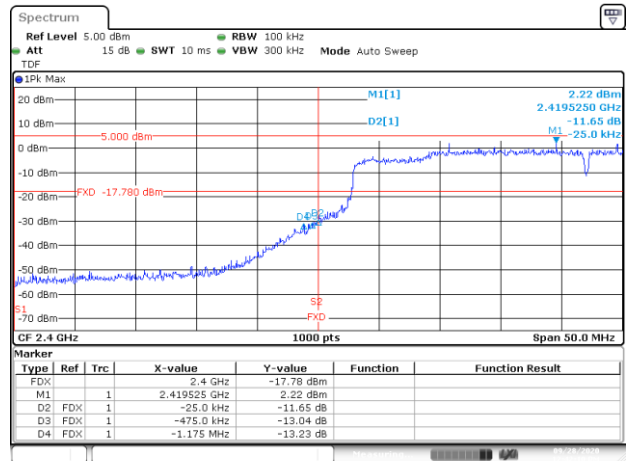
BE-NR, MIMO-B, 802.11ax40-HE0, Ch1
