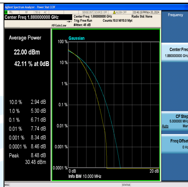
Band2-10MHz-16QAM-18900-50RB#0-PASS
