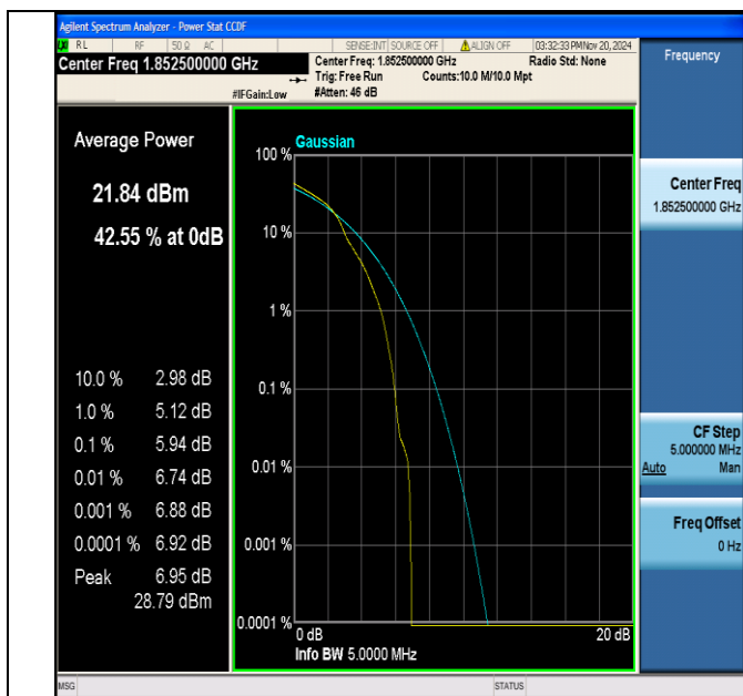
Band2-5MHz-16QAM-18625-1RB#0-PASS
