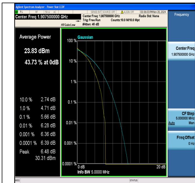
Band2-5MHz-QPSK-19175-1RB#0-PASS
