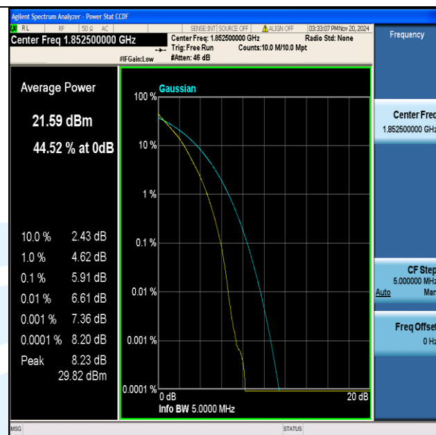
Band2-5MHz-QPSK-18625-25RB#0-PASS
