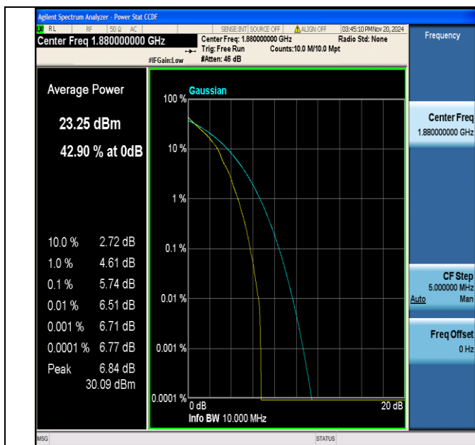
Band2-10MHz-QPSK-18900-1RB#0-PASS
