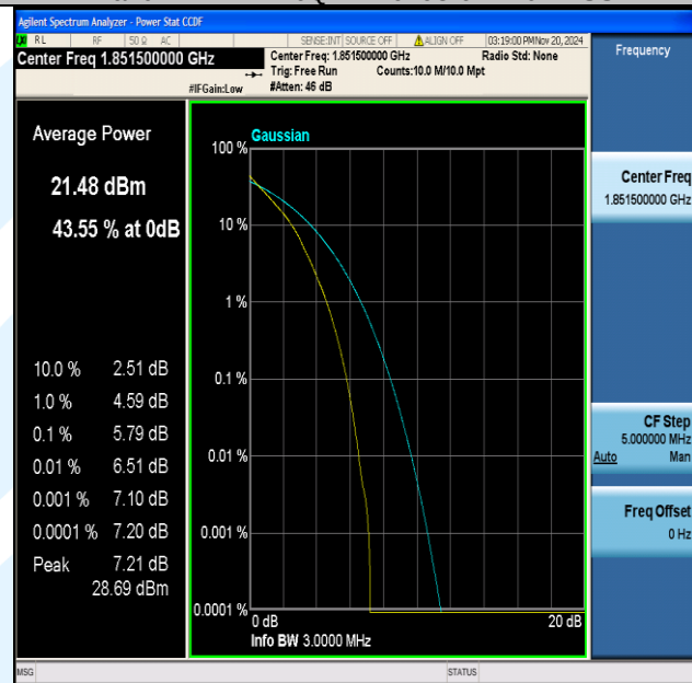
Band2-3MHz-QPSK-18615-15RB#0-PASS
