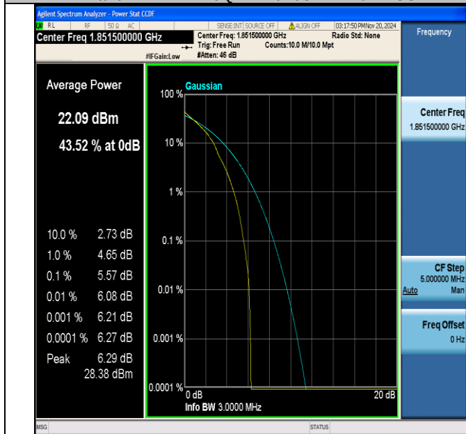
Band2-3MHz-QPSK-18615-1RB#0-PASS
