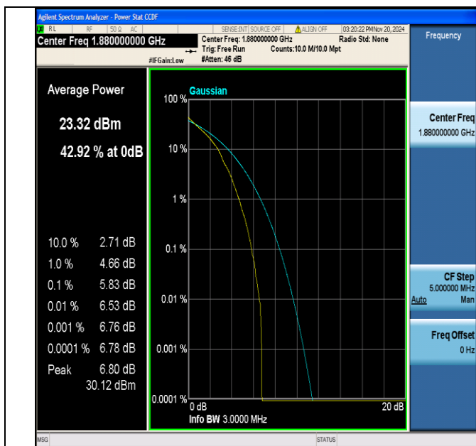
Band2-3MHz-QPSK-18900-1RB#0-PASS
