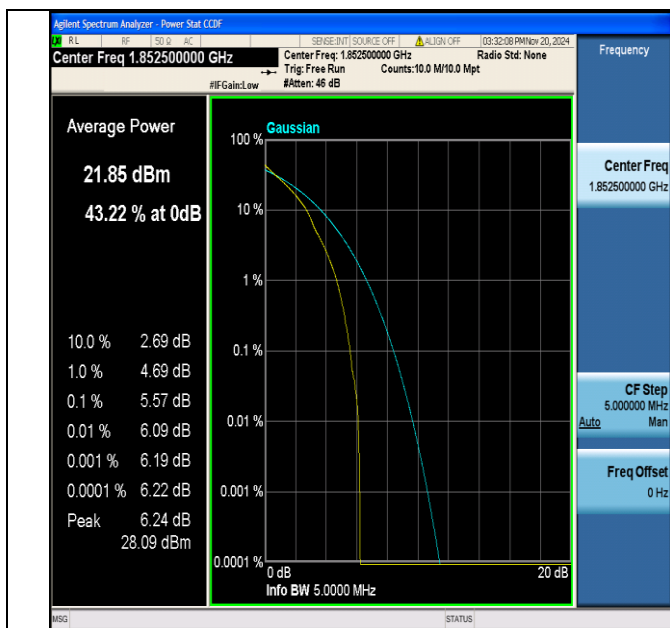
Band2-5MHz-QPSK-18625-1RB#0-PASS
