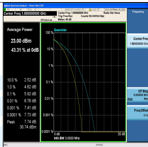
Band2-3MHz-QPSK-18900-15RB#0-PASS
