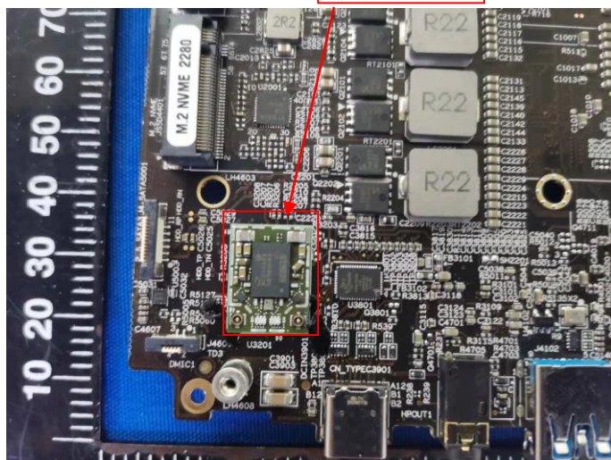
RF Module
