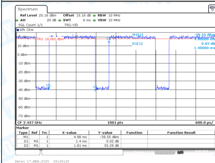
NTNV-11G-Ant1-2437
