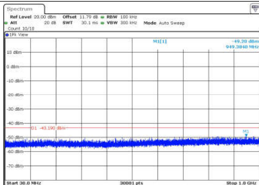
11G-Ant1-2462-30~1000-PASS
