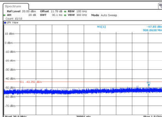
11G-Ant1-2437-30~1000-PASS
