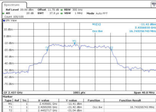
11G-Ant1-2437
