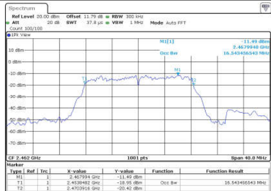
11G-Ant1-2462
