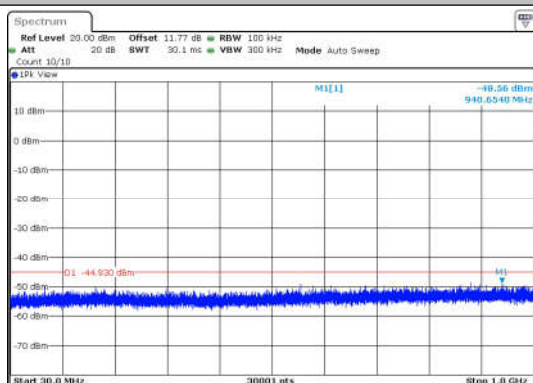
11G-Ant1-2412-30~1000-PASS
