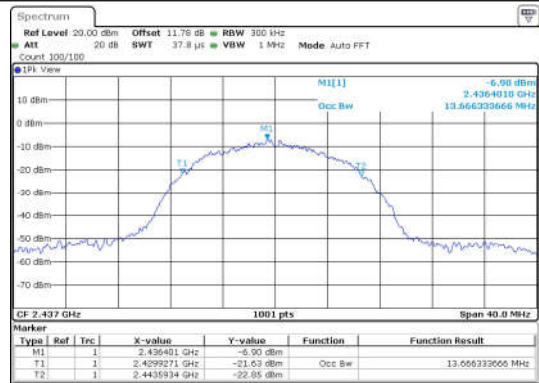
11B-Ant1-2437
