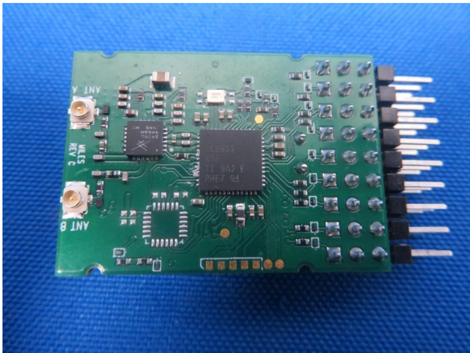
(4) EUT Photo
