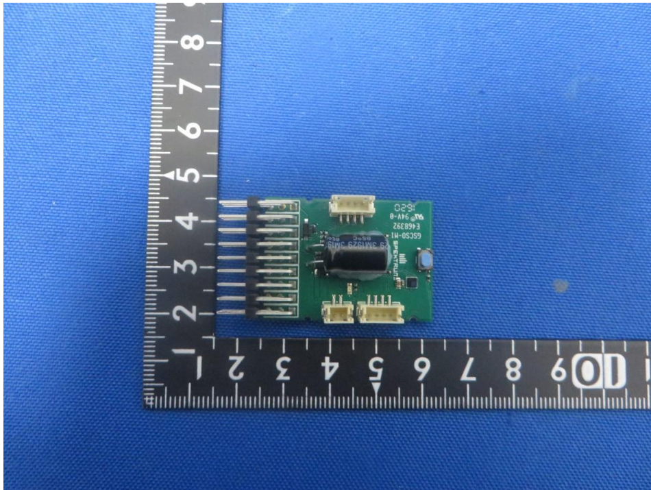
(3) EUT Photo
