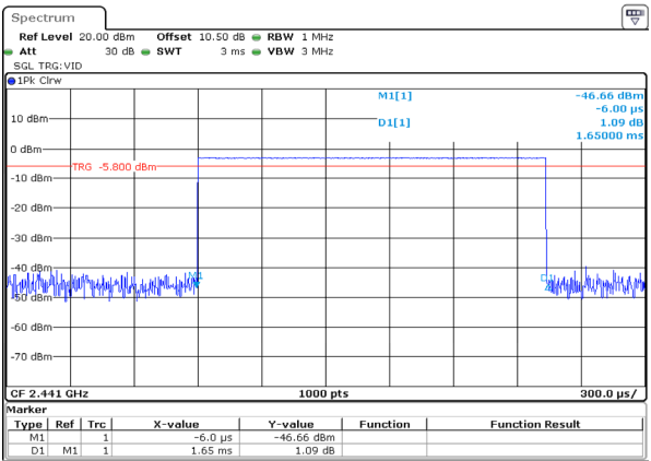
GFSK_Hopping_DH3 1.650ms
