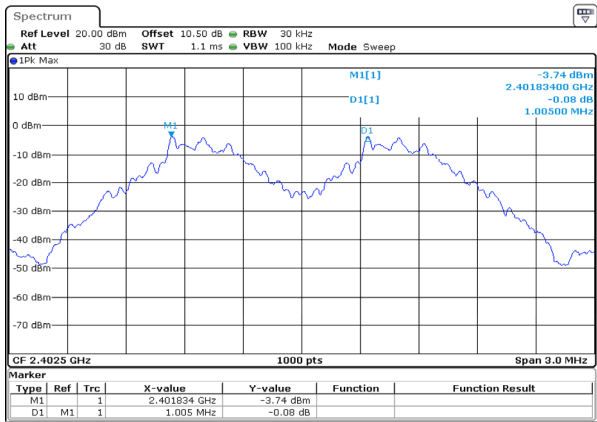
GFSK_Low 1.005MHz
