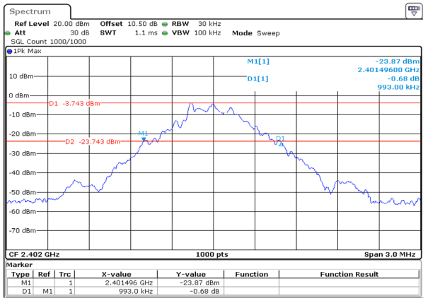
GFSK_Low 0.993MHz
