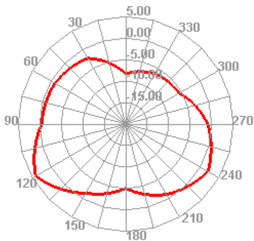
2.4G phi=0deg
