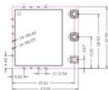
模组俯视图
