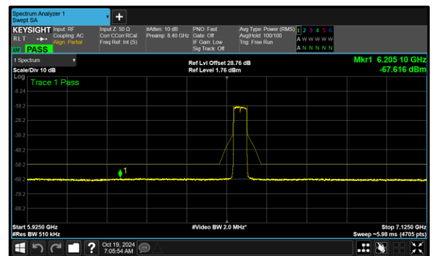
Figure 346 - A (Core 0) 802.11ax HE40 SU VLP 6565 MHz (CH123)
