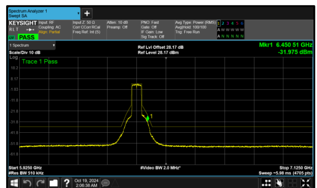
Figure 339 - A (Core 0) 802.11ax HE40 SU SP 6405 MHz (CH91)
