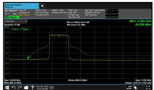
Figure 348 - A (Core 0) 802.11ax HE160 SU VLP 6345 MHz (CH79)
