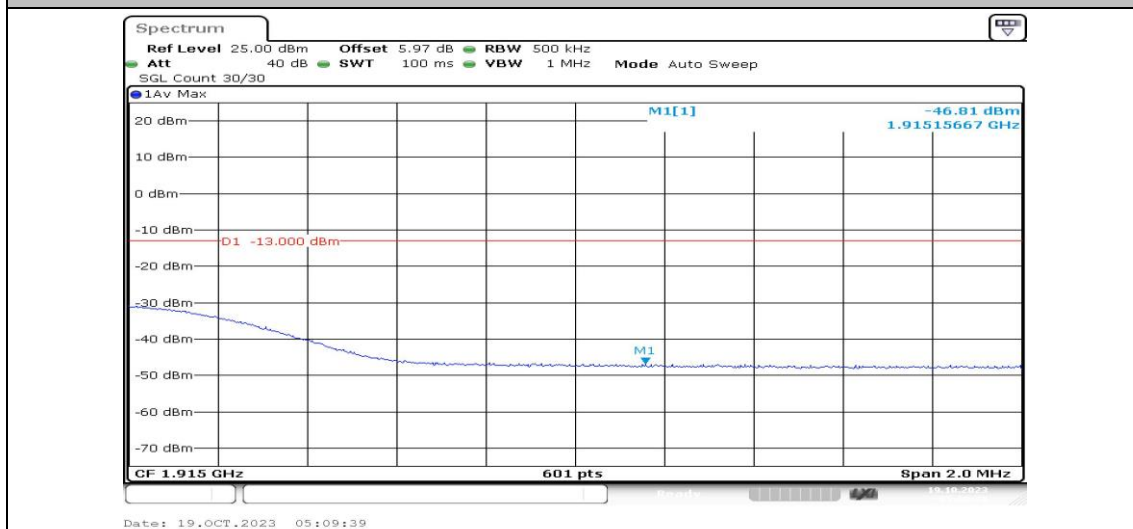
Band25-20MHz-QPSK-26590-1RB#0-PASS
