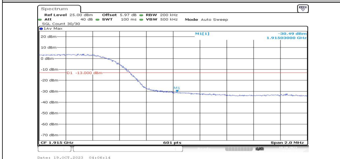
Band25-10MHz-QPSK-26640-50RB#0-PASS
