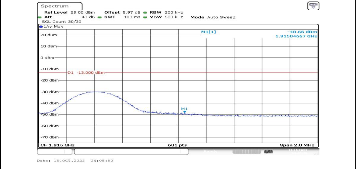
Band25-10MHz-QPSK-26640-1RB#0-PASS
