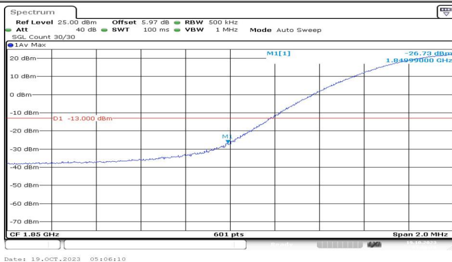
Band25-20MHz-QPSK-26140-1RB#0-PASS
