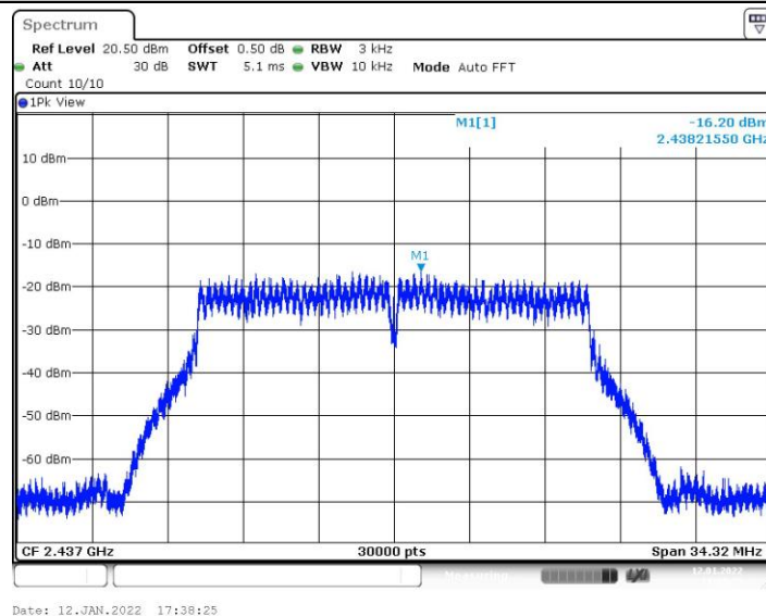
11N20MIMO_Ant8_2437
