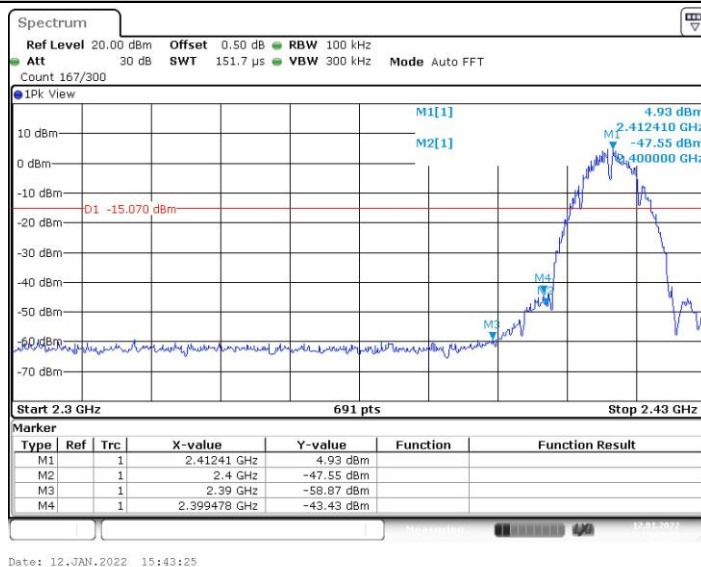
11B_Ant9_Low_2412
