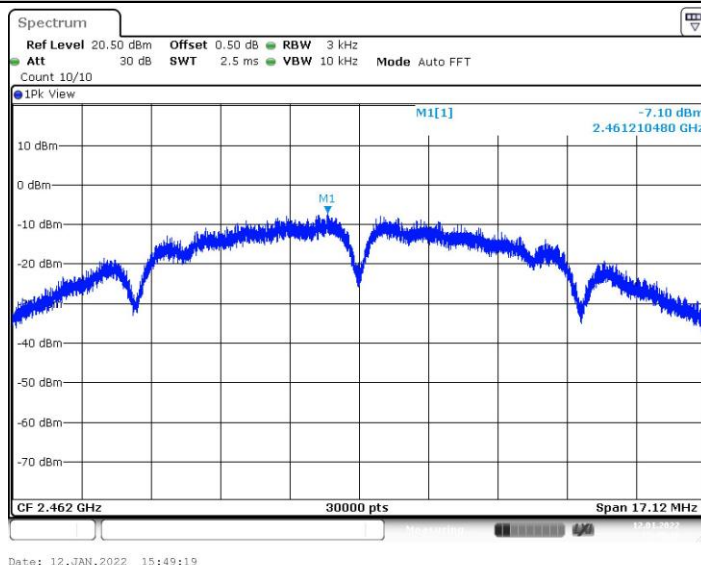
11B_Ant8_2462
