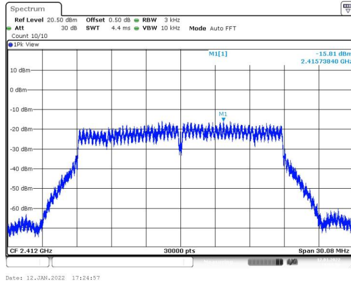
11N20MIMO_Ant9_2412
