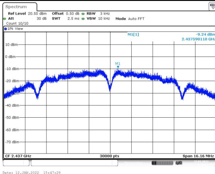
11B_Ant9_2437
