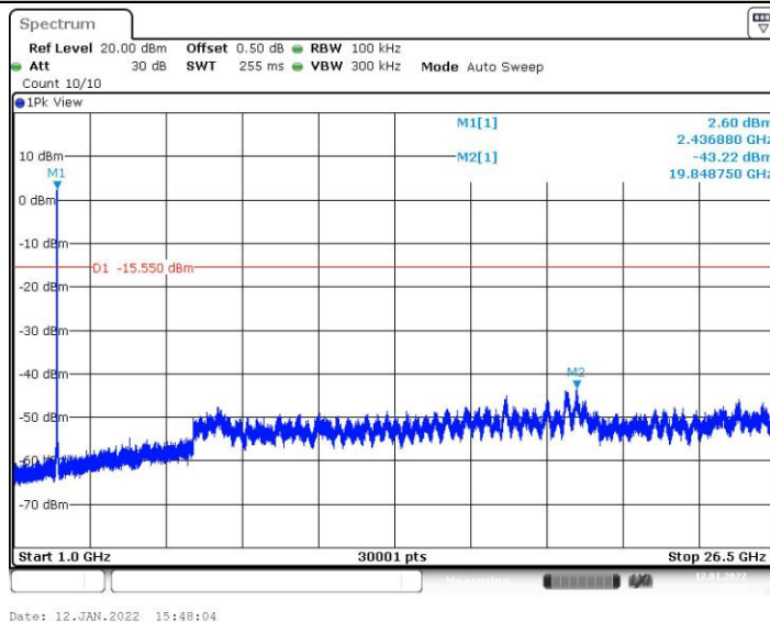
11B_Ant9_2437_0~Reference
