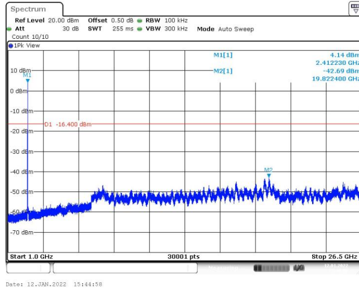
11B_Ant9_2412_0~Reference
