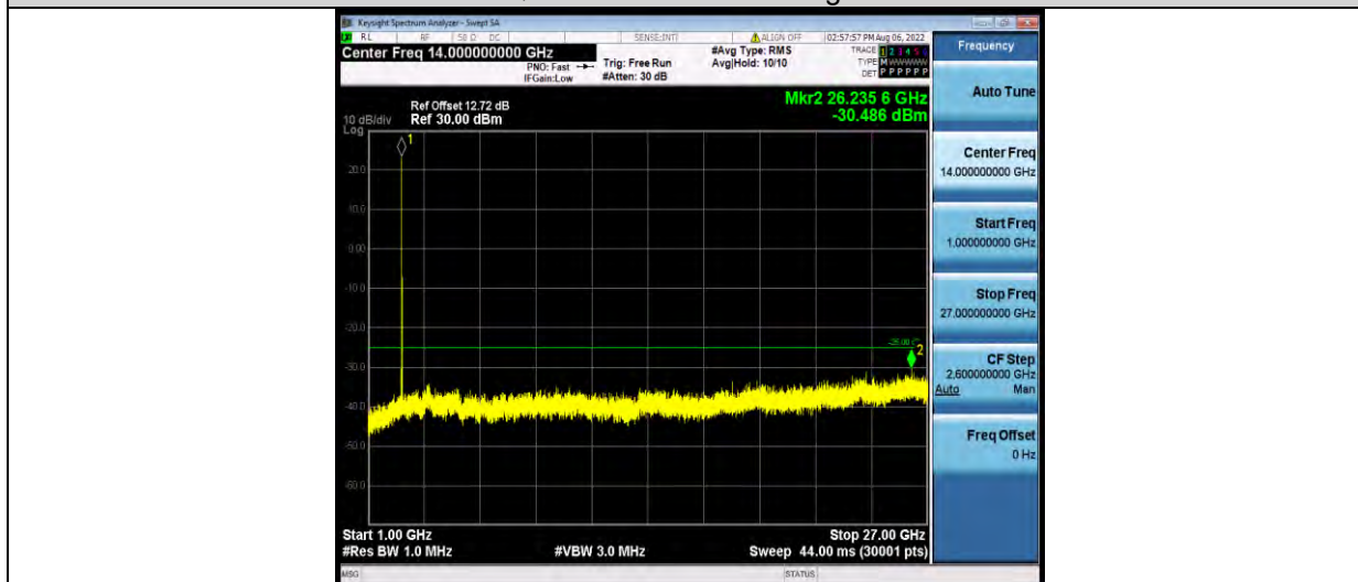
Band7-20MHz-64QAM-21350-1RB#0-Range2:1000~27000MHz
