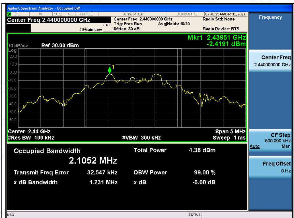
Test_Graph_FSK_ANT1_2440_DTSBW
