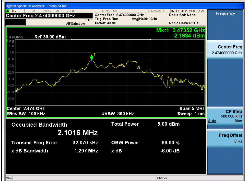
Test_Graph_FSK_ANT1_2474_DTSBW
