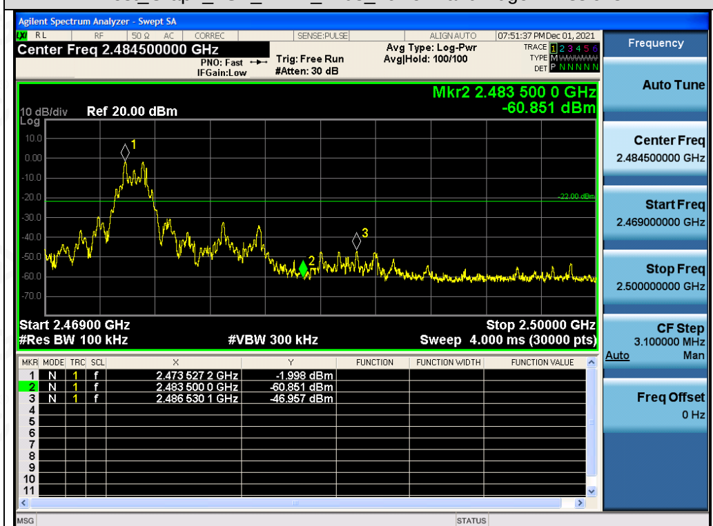
Test_Graph_FSK_ANT1_2474_Higher Band Edge Emissions
