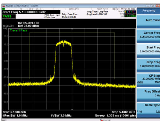
U-NII-1 ,802.11ax-HE40, 5230MHz, Ant3
