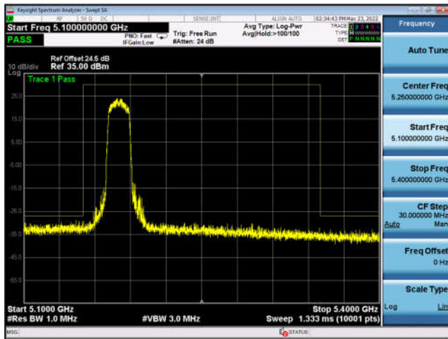
U-NII-1 ,802.11ax-HE20, 5220MHz, Ant3
