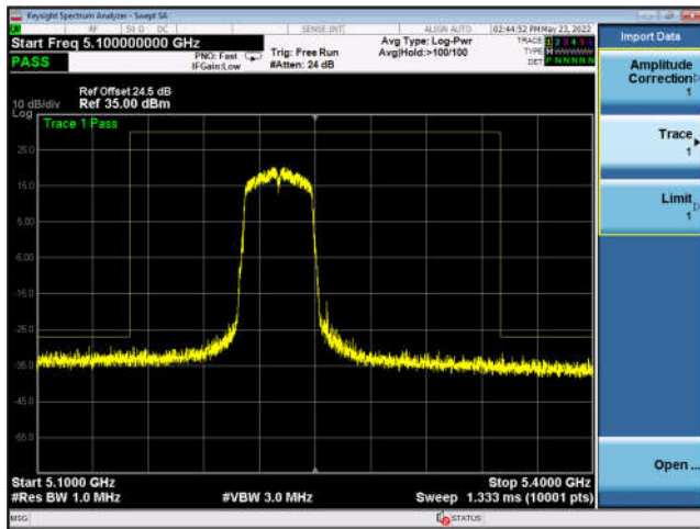
U-NII-1 ,802.11ax-HE40, 5190MHz, Ant3
