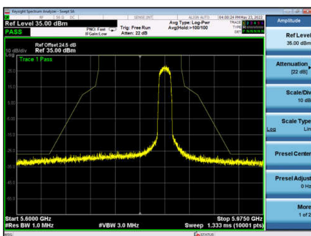
U-NII-3 ,802.11ax-HE20, 5825MHz, Ant0
