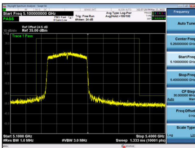
U-NII-1 ,802.11ax-HE80, 5210MHz, Ant3
