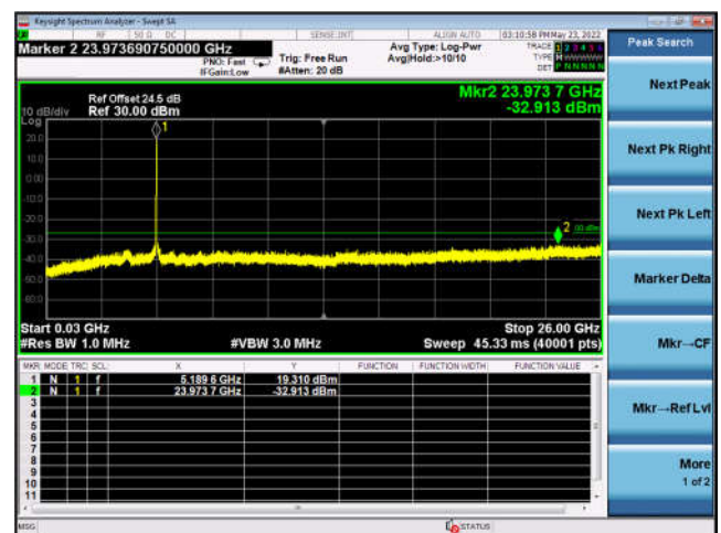
U-NII-1 ,802.11ax-HE40, 5230MHz, Ant1
