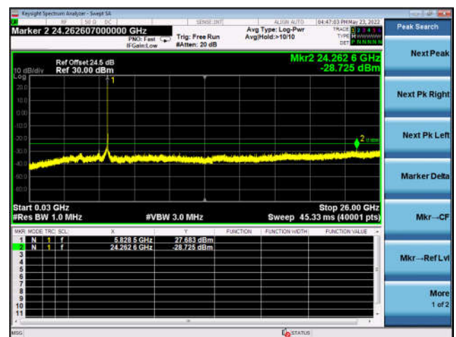
U-NII-3 ,802.11a, 5825MHz, Ant0
