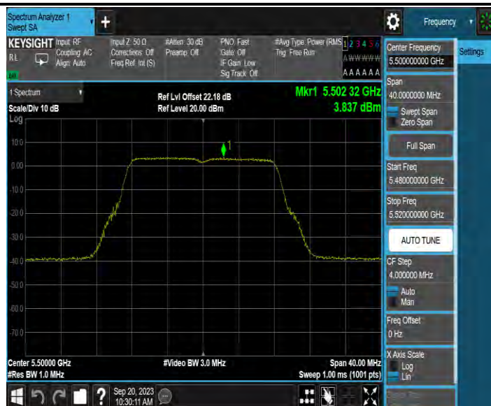
11A-MIMO_Ant4_5500
