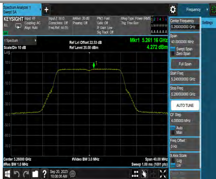
11A-MIMO_Ant3_5260
