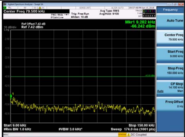
20MHz_LCH_QPSK_1RB#0
