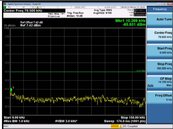
20MHz_LCH_QPSK_1RB#0
