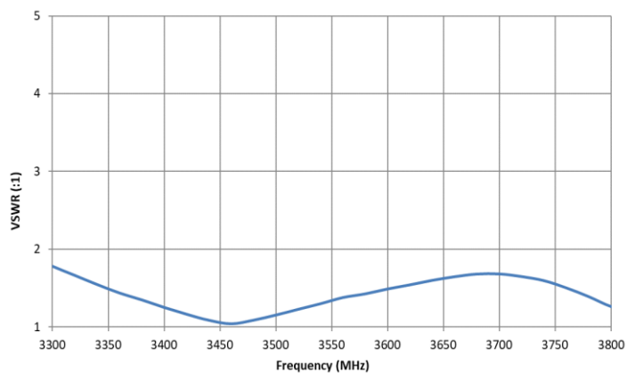
VSWR
