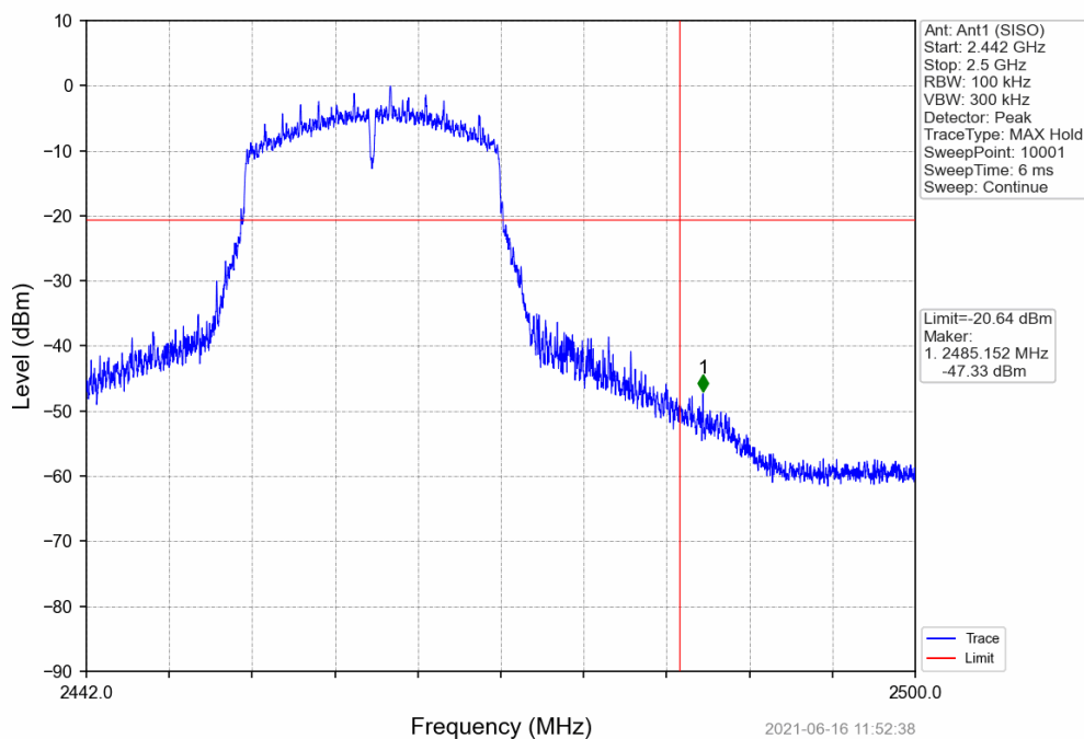
802.11n(HT20)_HCH_2462MHz_Ant1 (SISO)_NTNV
