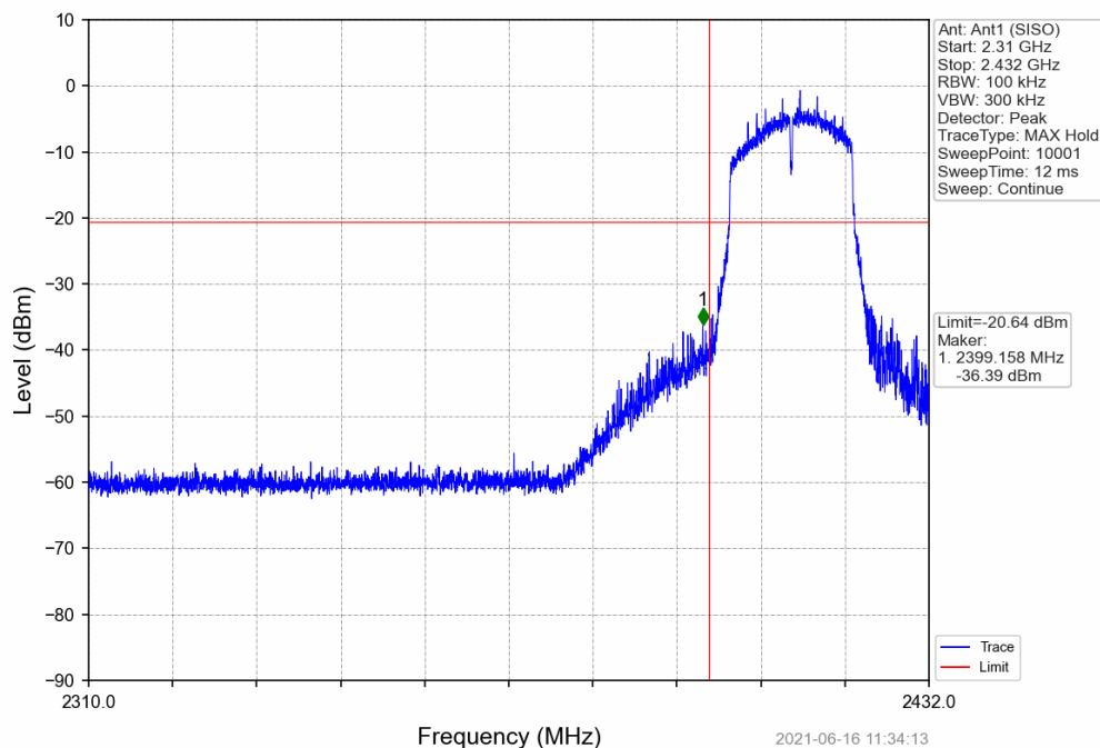
802.11n(HT20)_LCH_2412MHz_Ant1 (SISO)_NTNV
