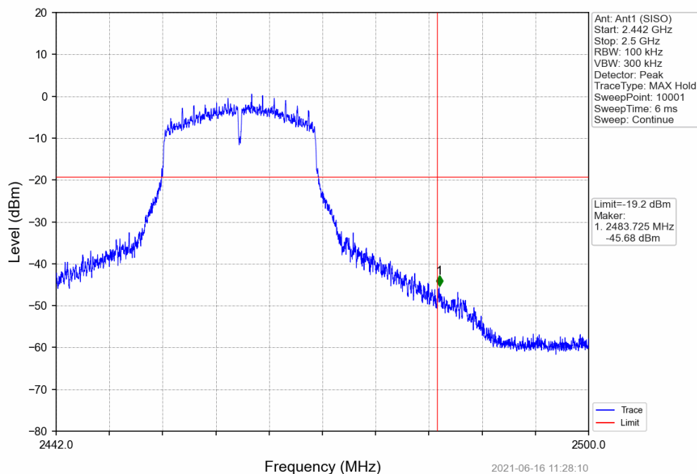
802.11g_HCH_2462MHz_Ant1 (SISO)_NTNV
