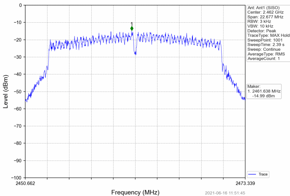
802.11n(HT20)_HCH_2462MHz_Ant1 (SISO)_NTNV
