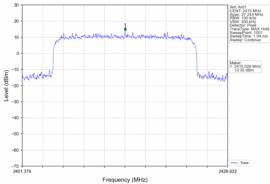
Slot20_LCH_2415MHz_Ant1_NTNV
