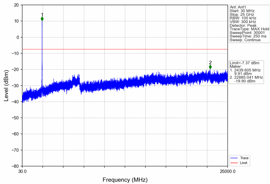
Slot20_MCH_2440MHz_Ant1_NTNV
