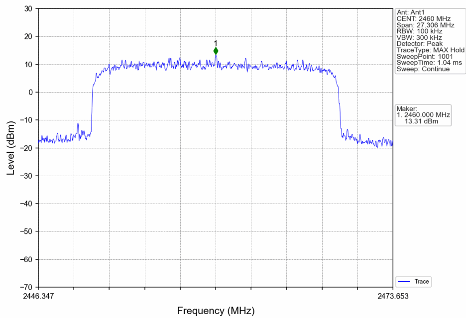
Slot20_HCH_2460MHz_Ant1_NTNV
