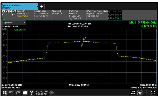
SP1-C0 5755 MHz (CH151)
