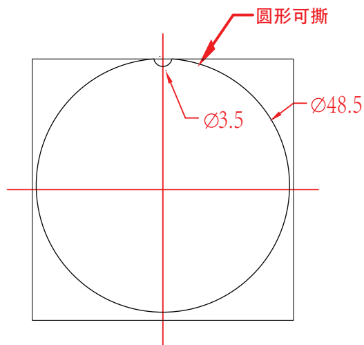
标贴尺寸图
