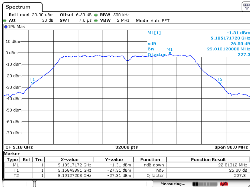
26dB BW 802.11a Channel: 36
