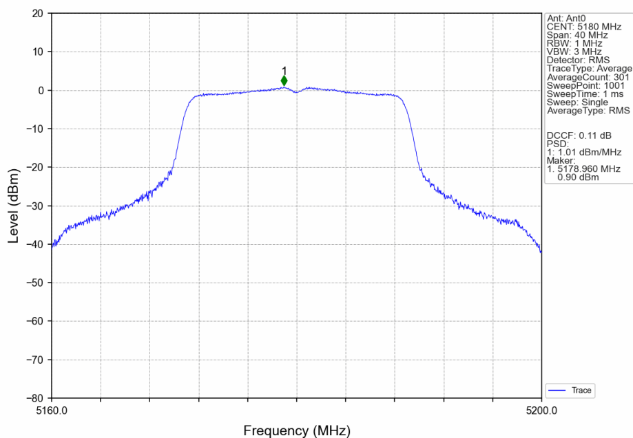
802.11n(HT20)_LCH_5180MHz_Ant0_NTNV
