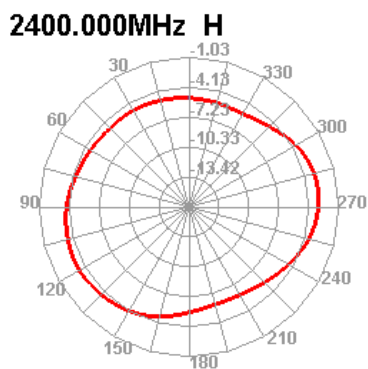
2D 增益模式 2D Gain Pattern (2400 MHz)
