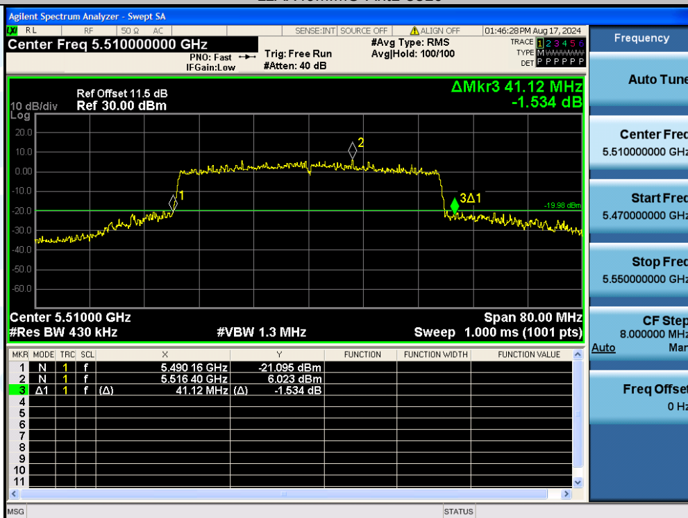
11AX40MIMO-Ant2-5510
