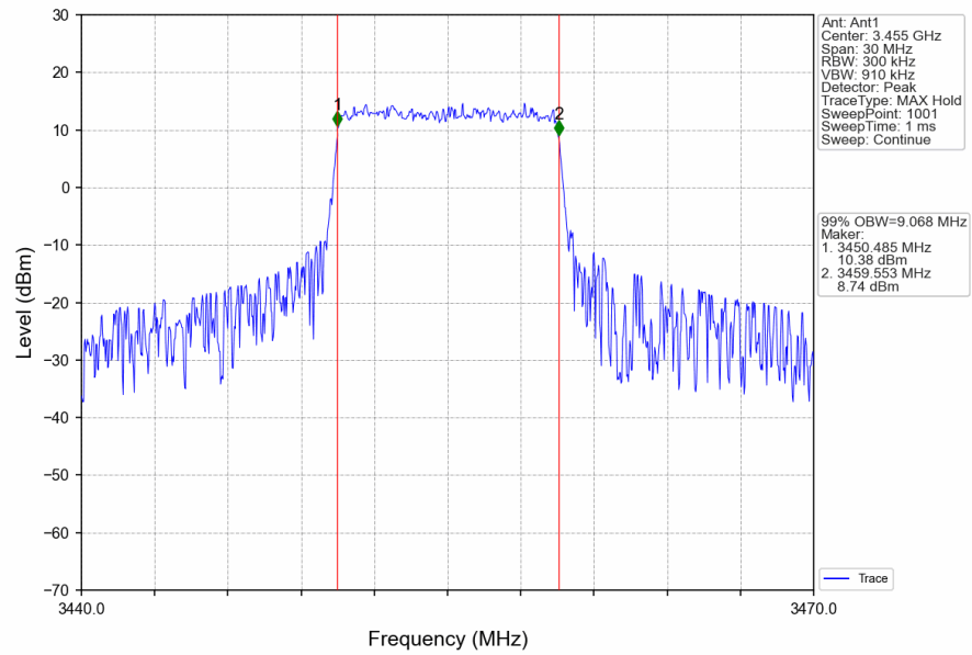
Band42a_10MHz_16QAM_LCH_3455MHz_RB_50_0_NTNV
