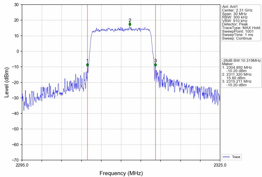
Band40a_10MHz_16QAM_LCH_2310MHz_RB_50_0_NTNV
