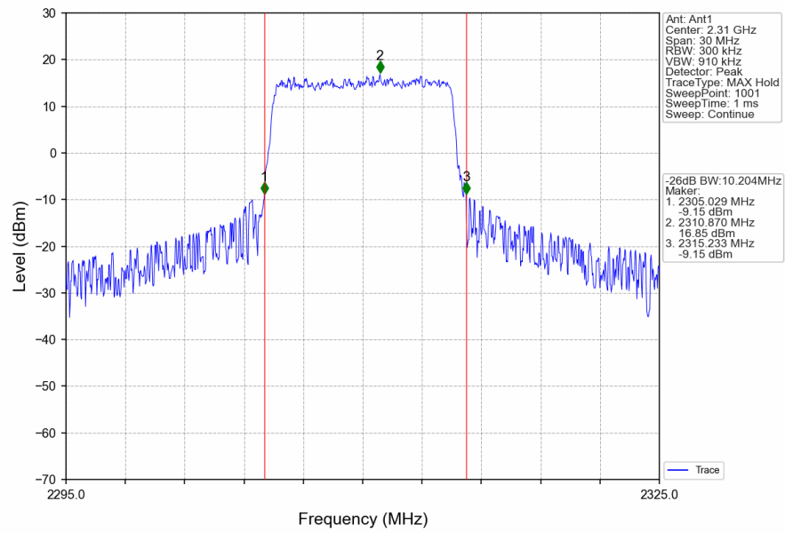
Band40a_10MHz_16QAM_LCH_2310MHz_RB_50_0_NTNV
