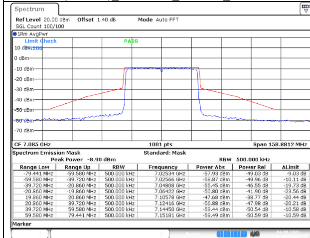
802.11ax (40MHz) 7085MHz Chain A NSS-4
