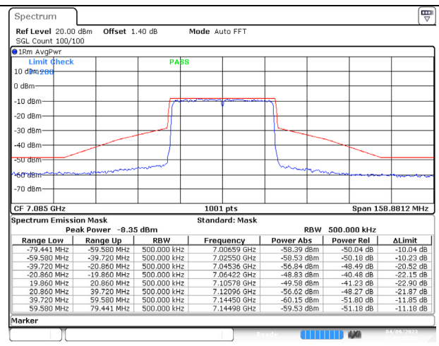
802.11ax (40MHz) 7085MHz Chain D NSS-4
