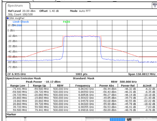
802.11ax (40MHz) 6925MHz Chain C NSS-4
