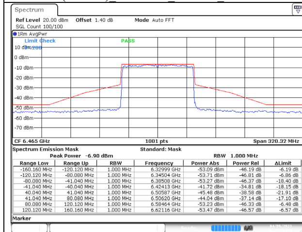
802.11ax (80MHz) 6465MHz Chain C NSS-4
