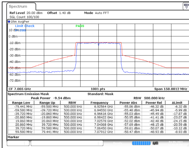
802.11ax (40MHz) 7005MHz Chain A NSS-4
