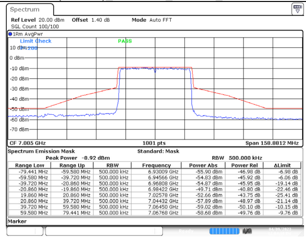
802.11ax (40MHz) 7005MHz Chain D NSS-4
