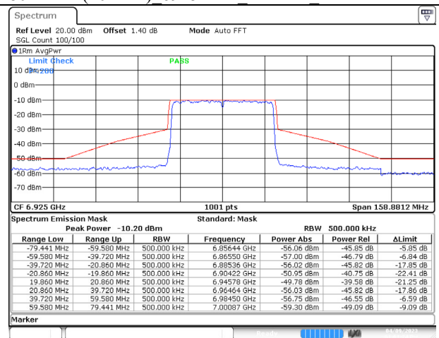
802.11ax (40MHz) 6925MHz Chain D NSS-4
