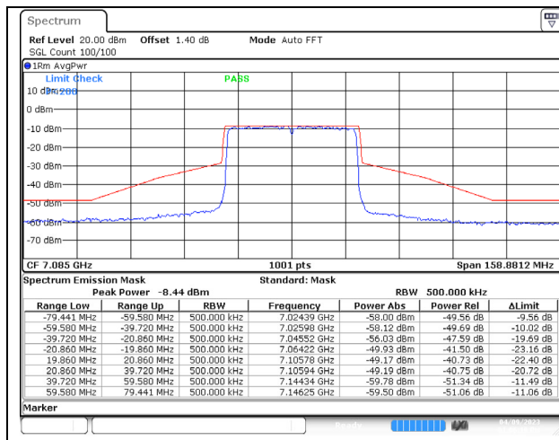
802.11ax (40MHz) 7085MHz Chain C NSS-4
