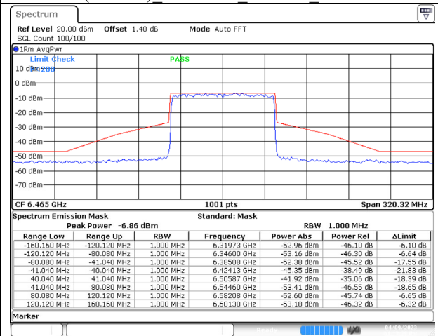
802.11ax (80MHz) 6465MHz Chain D NSS-4
