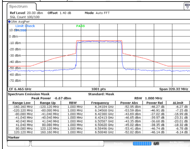
802.11ax (80MHz) 6465MHz Chain A NSS-4
