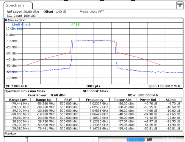
802.11ax (40MHz) 7085MHz Chain B NSS-4
