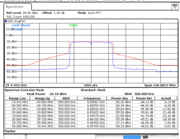
802.11ax (40MHz) 6925MHz Chain B NSS-4
