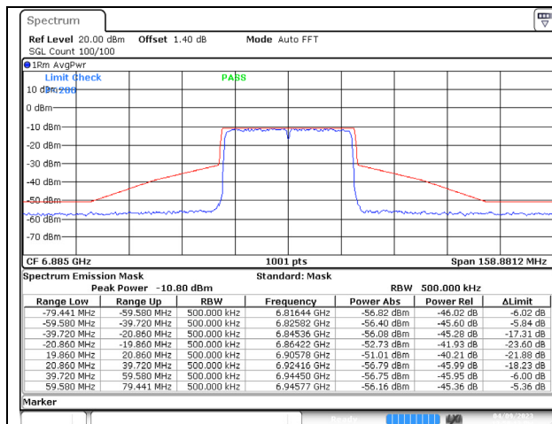
802.11ax (40MHz) 6885MHz Chain C NSS-4
