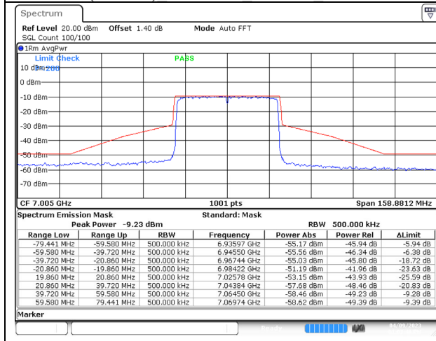
802.11ax (40MHz) 7005MHz Chain C NSS-4
