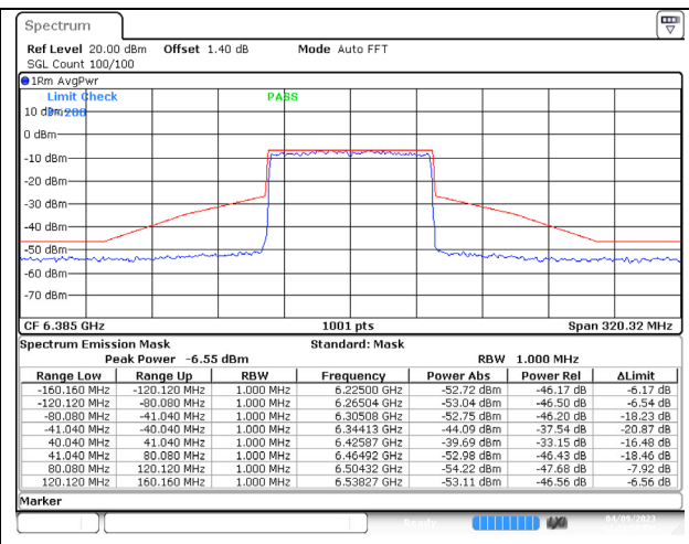
802.11ax (80MHz) 6385MHz Chain D NSS-4
