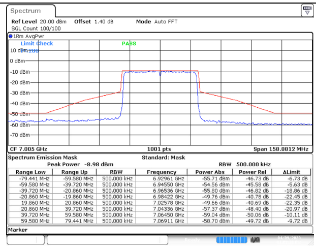
802.11ax (40MHz) 7005MHz Chain B NSS-4
