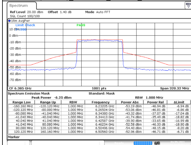
802.11ax (80MHz) 6385MHz Chain A NSS-4
