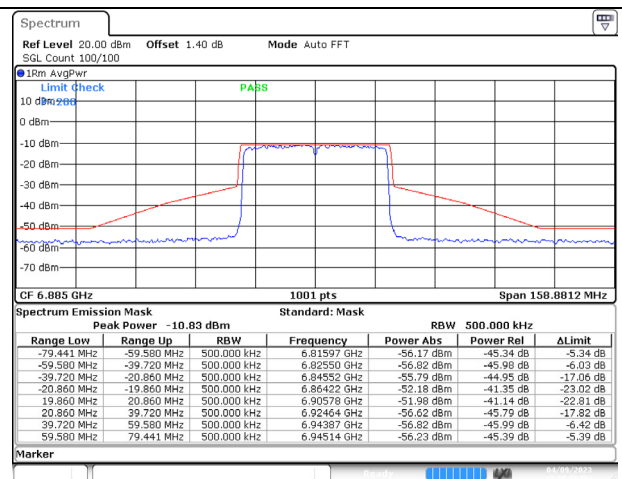
802.11ax (40MHz) 6885MHz Chain D NSS-4
