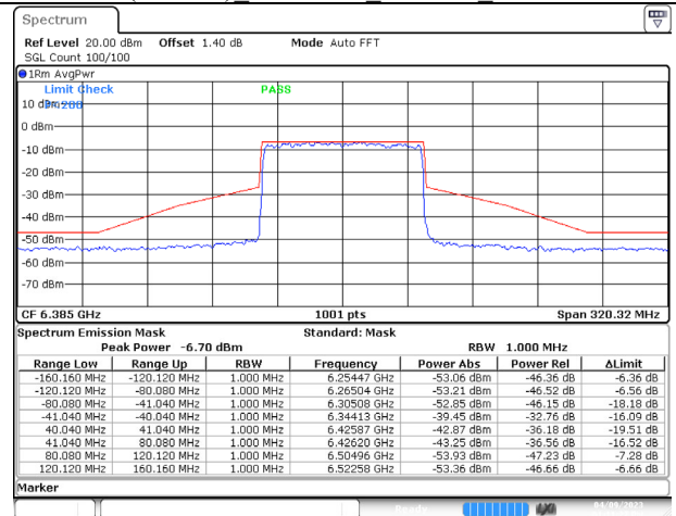
802.11ax (80MHz) 6385MHz Chain B NSS-4
