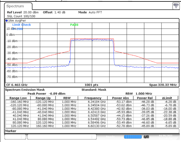
802.11ax (80MHz) 6465MHz Chain B NSS-4
