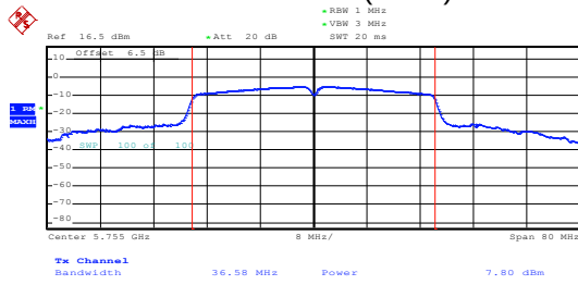
802.11ac(HT40)
